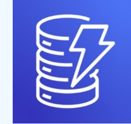
Amazon DynamoDB
